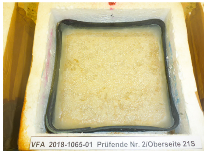
Prüfende Platte Nr. 2 Oberseite mit Finalit Nr. 21S Porenfüller behandelt, Abwitterungsmenge 8 \text{ g/m}^2 . Foto: Magistrat der Stadt Wien, Magistratsabteilung 39
